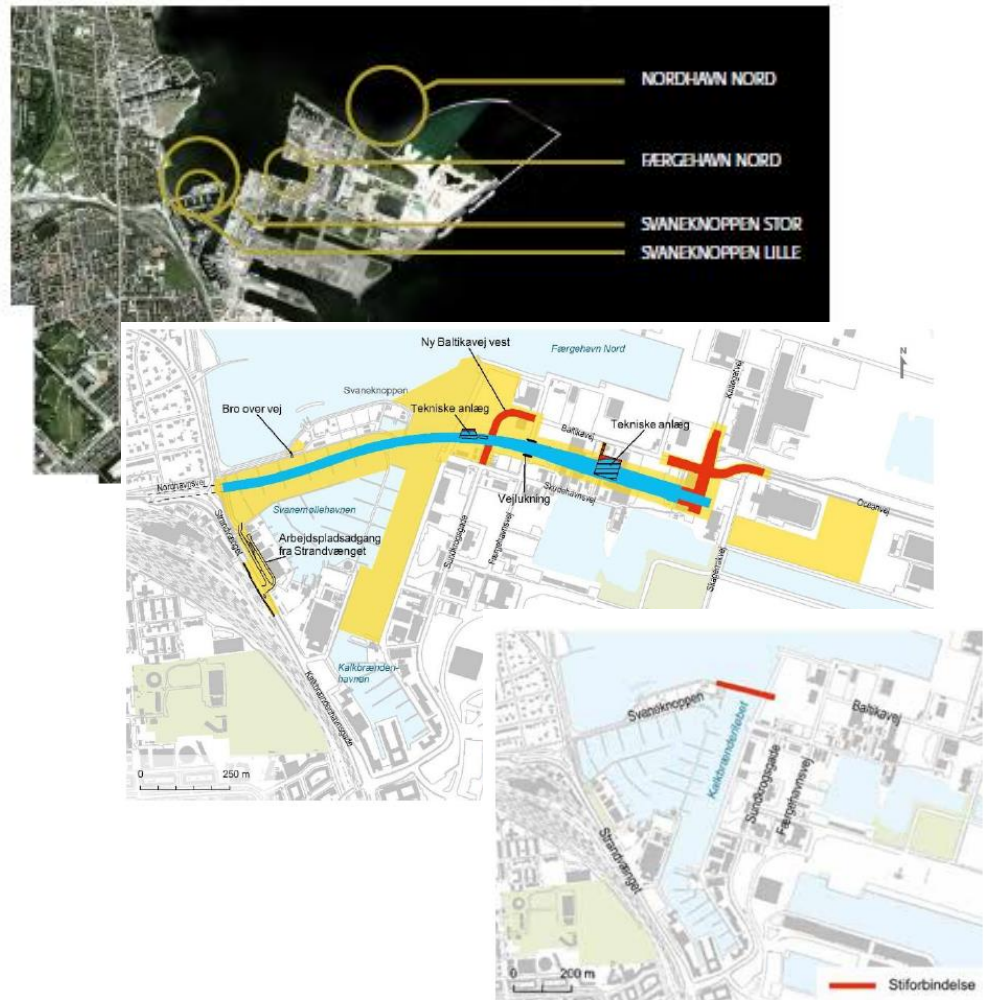
Figur 6.1 Linjeføring for stiforbindelse til fodgængere og cyklister mellem Svaneknoppen og Nordhavn.
